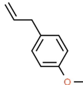
estragole
