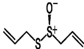
Allicin
